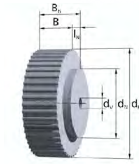
Lagerscheiben ab z = 48 ohne Bordscheiben
