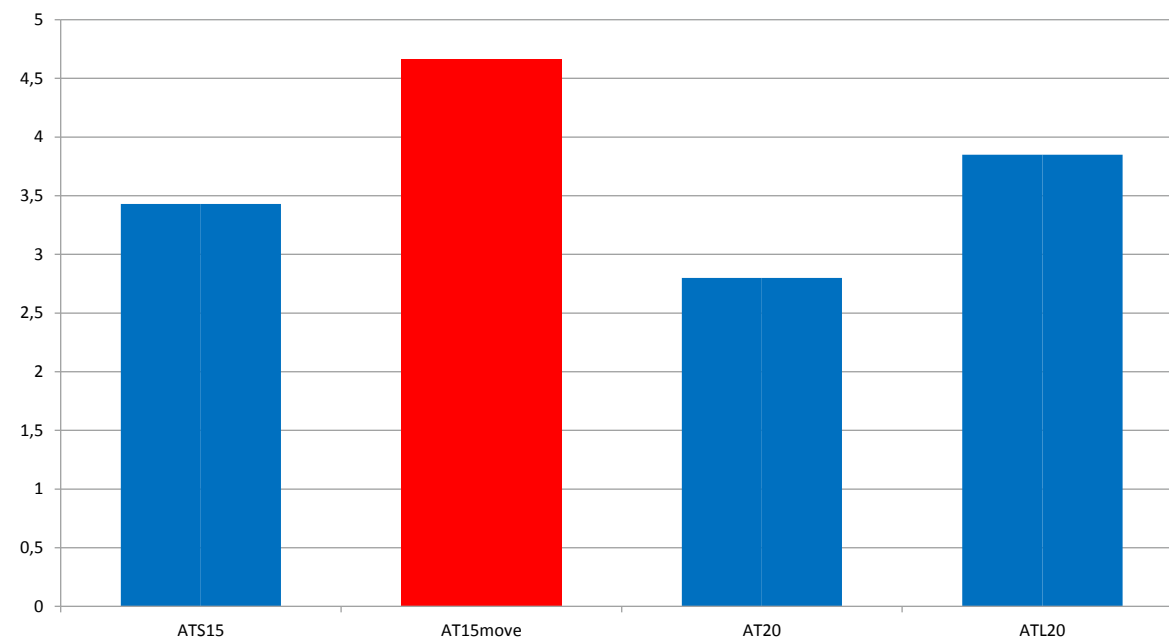
Spezifische Federrate in 10^6 N (Riemenbreite 50 mm, 0,4%-Grenze)
