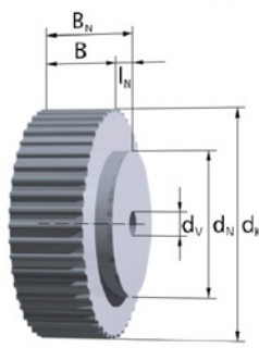
Lagerscheiben ab z = 44 ohne Bordscheiben
