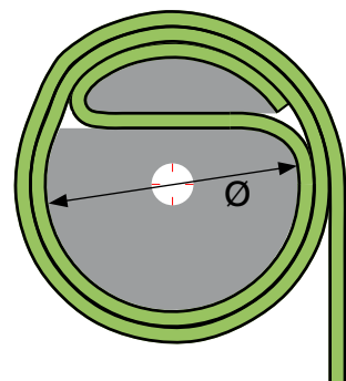
Endbefestigung Typ 2 (Prinzip-Darstellung)
